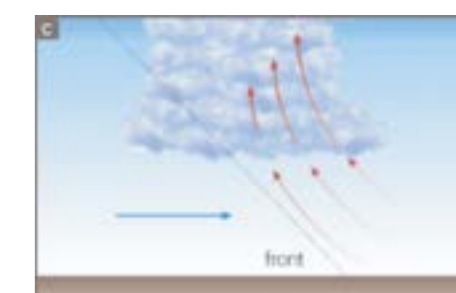
Precipitació frontal
