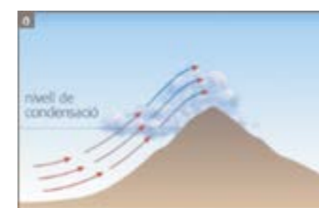
Precipitació orogràfica
