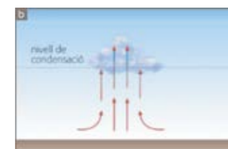
Precipitació conectiva
